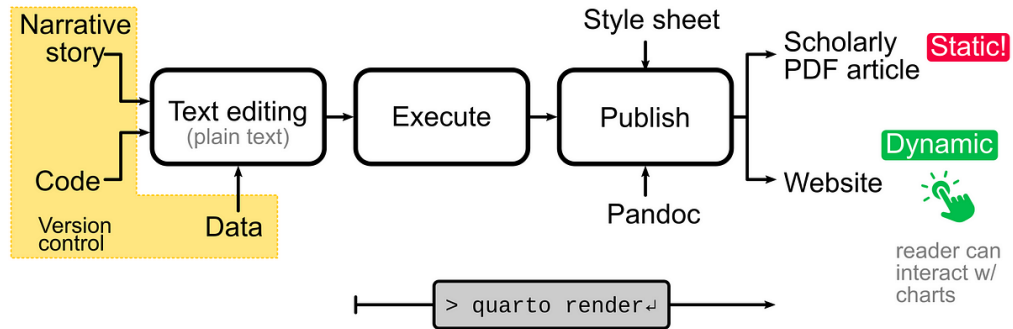
Figura 6.4: Workflow de uma pesquisa empírica utilizando Quarto
