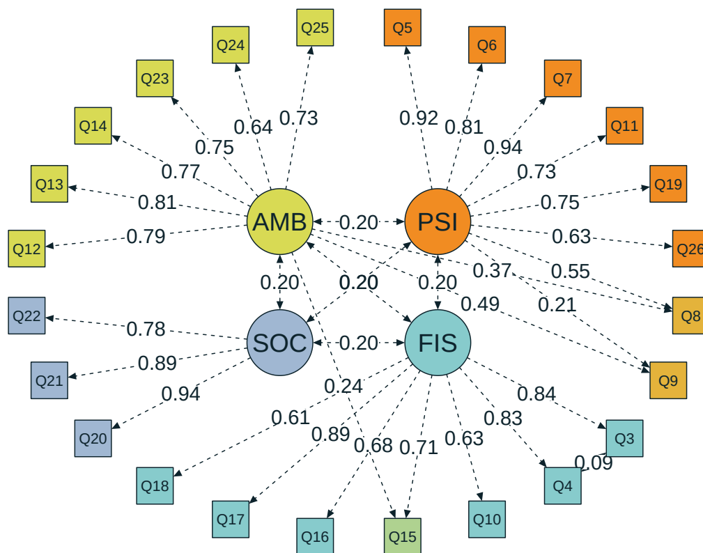
Figura 2: Modelo de quatro fatores correlacionados com covariância residual Q3–Q4 e três cargas cruzadas. Nota. PSI = psicológico; FIS = físico; SOC = relações sociais; AMB = ambiente. Mantém-se a estrutura do primeiro modelo e acrescentam-se as cargas do fator psicológico em Q8 e Q9 e do fator ambiental em Q15. A figura representa a especificação (cargas fixas) do modelo populacional alternativo. Ao estimarmos com parâmetros livres, as cargas e a covariância residual são ajustadas para a amostra, e temos nosso modelo alternativo ( H_1 )
