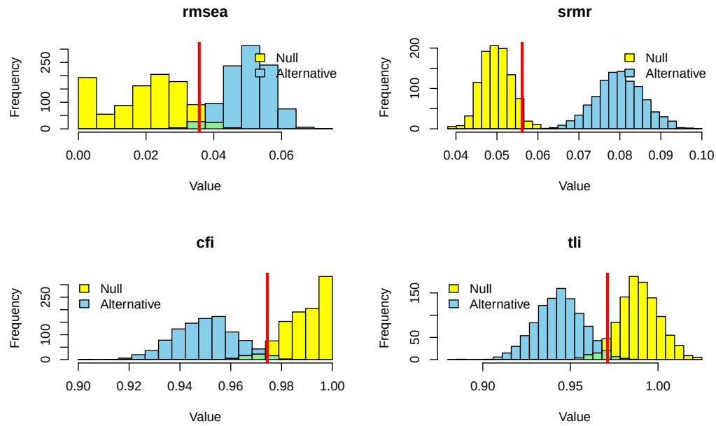
Figura 6: Distribuições empíricas dos índices de ajuste em 1.000 replicações com N = 200 .
