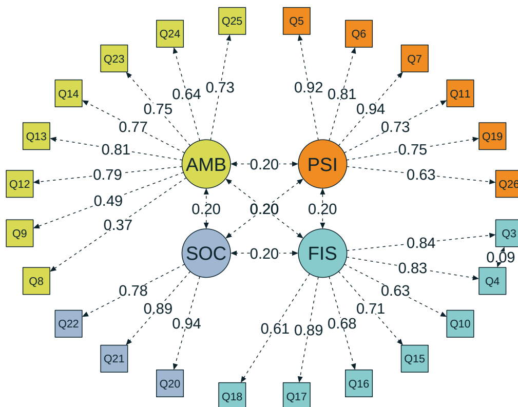
Figura 1: Modelo de quatro fatores correlacionados com covariância residual entre Q3 e Q4. Nota. PSI = psicológico; FIS = físico; SOC = relações sociais; AMB = ambiente. A figura representa a especificação (cargas fixas) do modelo populacional. Ao estimarmos com parâmetros livres, as cargas e a covariância residual são ajustadas para a amostra, e temos nosso modelo de análise ( H_0 )
