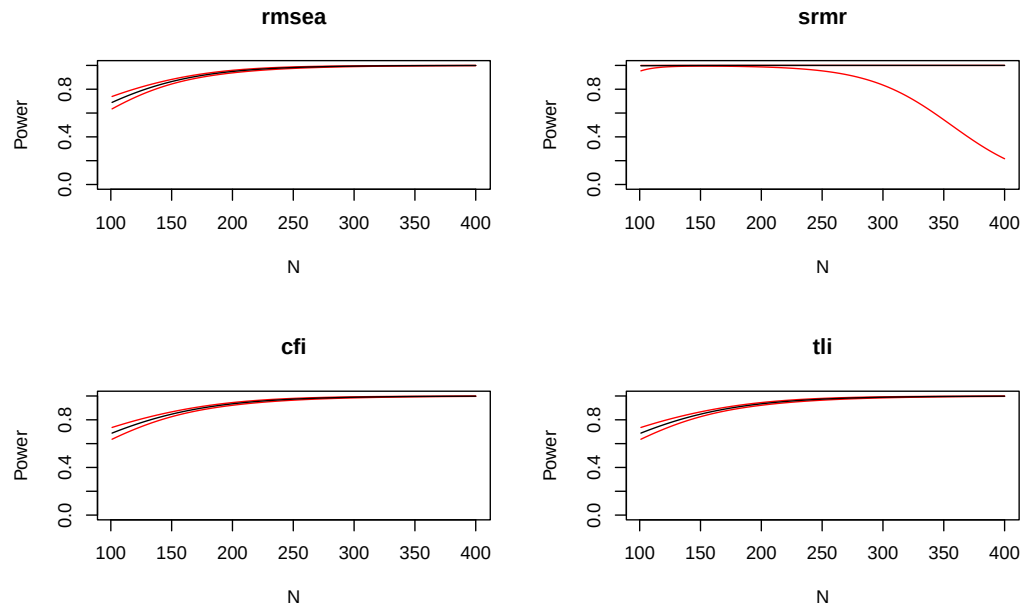
Figura 4: Curvas de poder com suavização logística sob não normalidade leve e 10% de dados ausentes MCAR.
