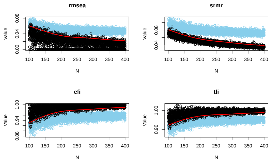
Figura 5: Poder empírico sem suavização logística sob não normalidade leve e 10% de dados ausentes MCAR.
