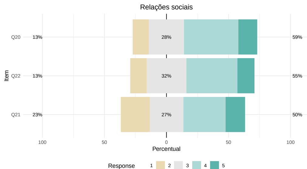
Figura 8: Distribuição das categorias de resposta Likert no construto Relações sociais.
