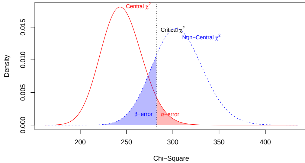
Figura 3: Distribuições central e não central do qui-quadrado na análise analítica de poder baseada nos modelos.
