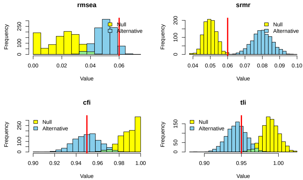
Figura 7: Distribuições dos índices de ajuste avaliadas por pontos de corte tradicionais em 1.000 replicações com N = 200 .
