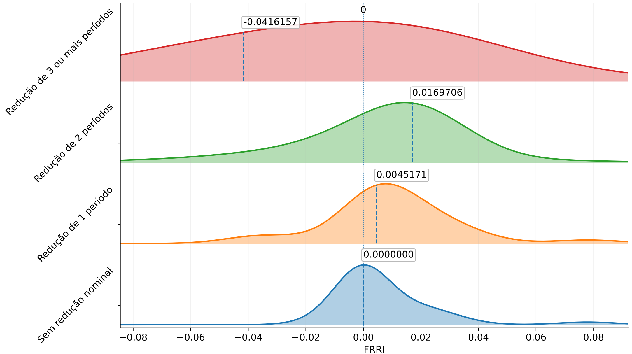
Distribuição do FRRl por ganho nominal de prazo Instância J3031_1
