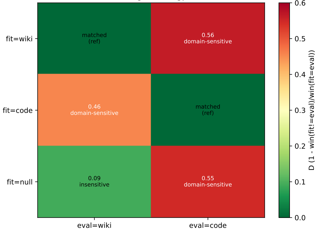
D matrix (budget=2.5, gpt2-scale)
