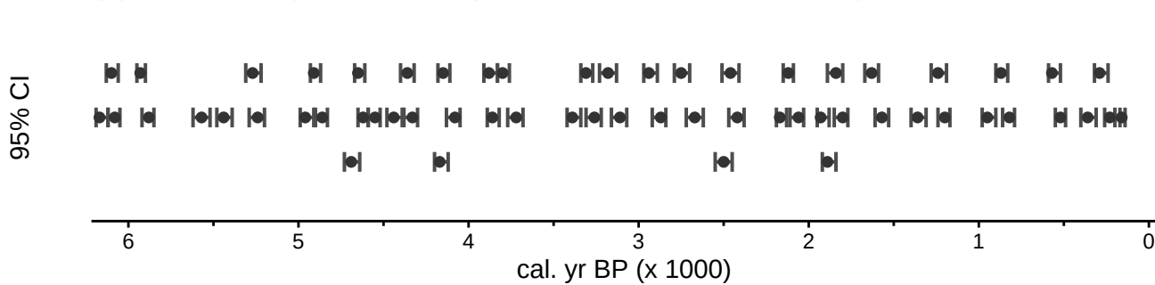
(d) 95% CI on peak timing (1000-chronology ensemble)
