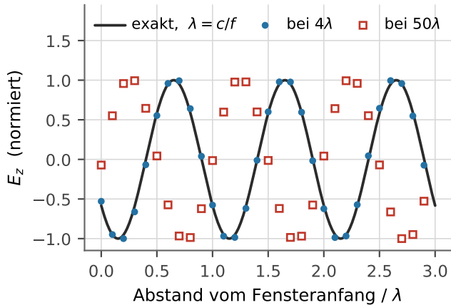
(b) Phasenlage nah und fern, N_\lambda = 10
