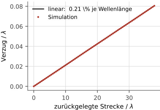
(a) Aufsummierter Verzug, N_\lambda = 20
