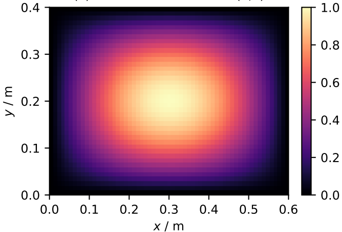
(a) Simulierte Grundmode (1,1)
