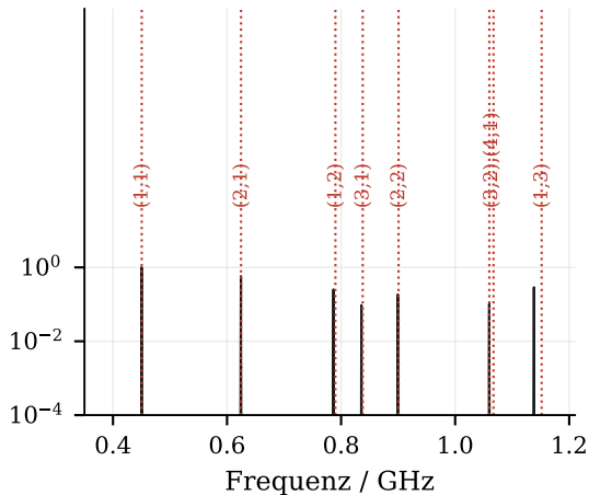
(a) Spektrum, punktiert die Vorhersage
