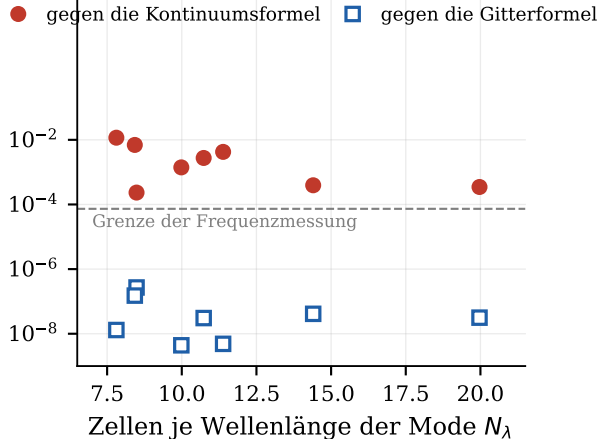
(b) Abweichung je Mode
