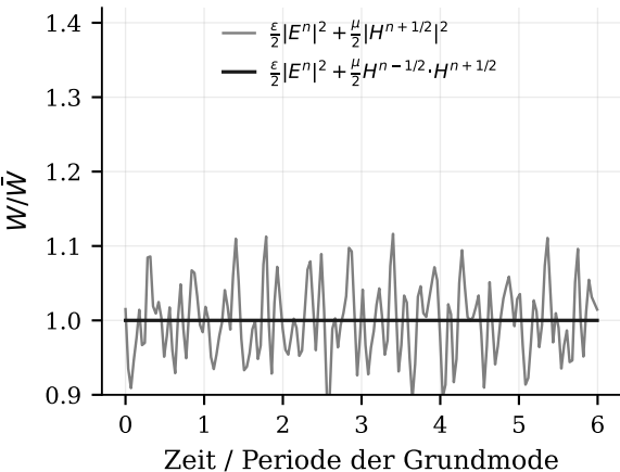
(a) Energie über der Zeit
