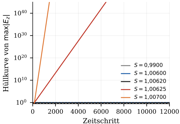
(b) Verhalten an der Stabilitätsgrenze
