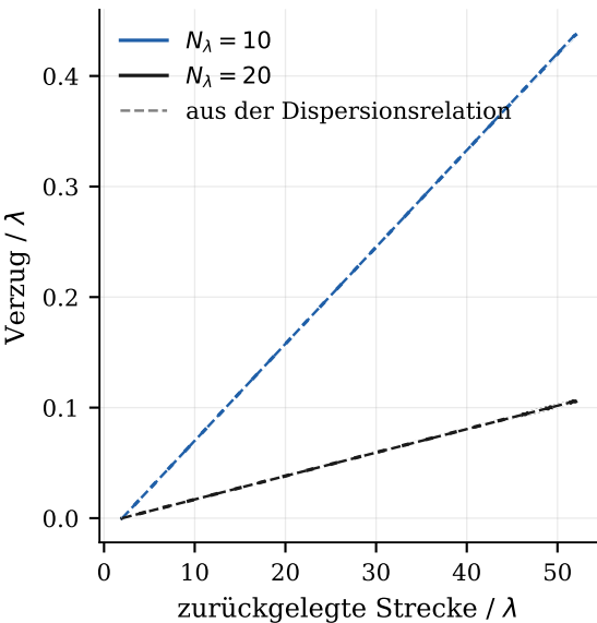
(a) Aufsummierung über die Laufstrecke
