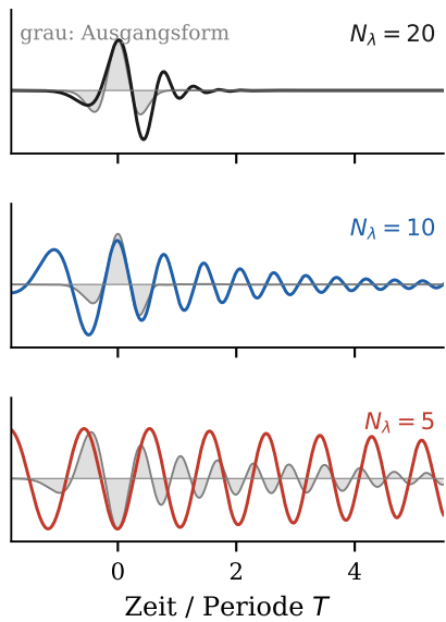
(b) Pulsform vor und nach 36 \lambda
