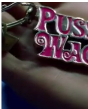
13 Kill Bill
