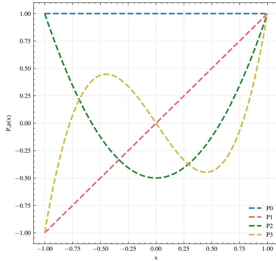
SciPy Implementation (Legendre)
