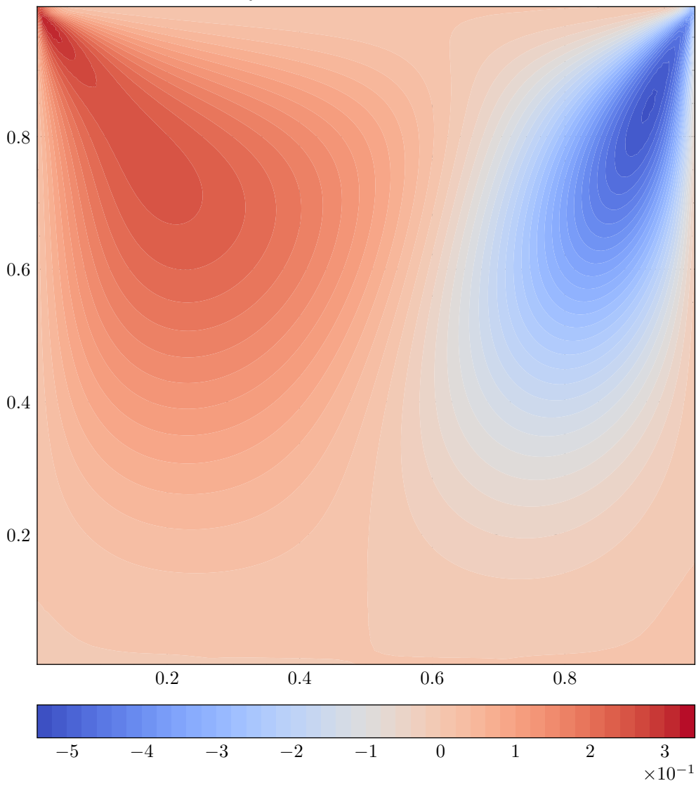
v-velocity — Simulation ID: 5e7591a2
