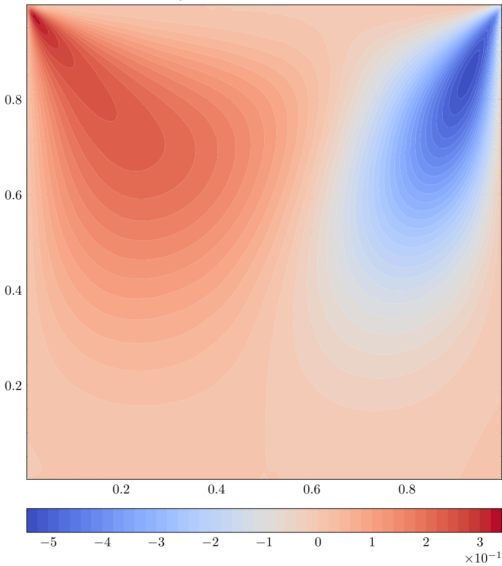
v-velocity — Simulation ID: a0579211
