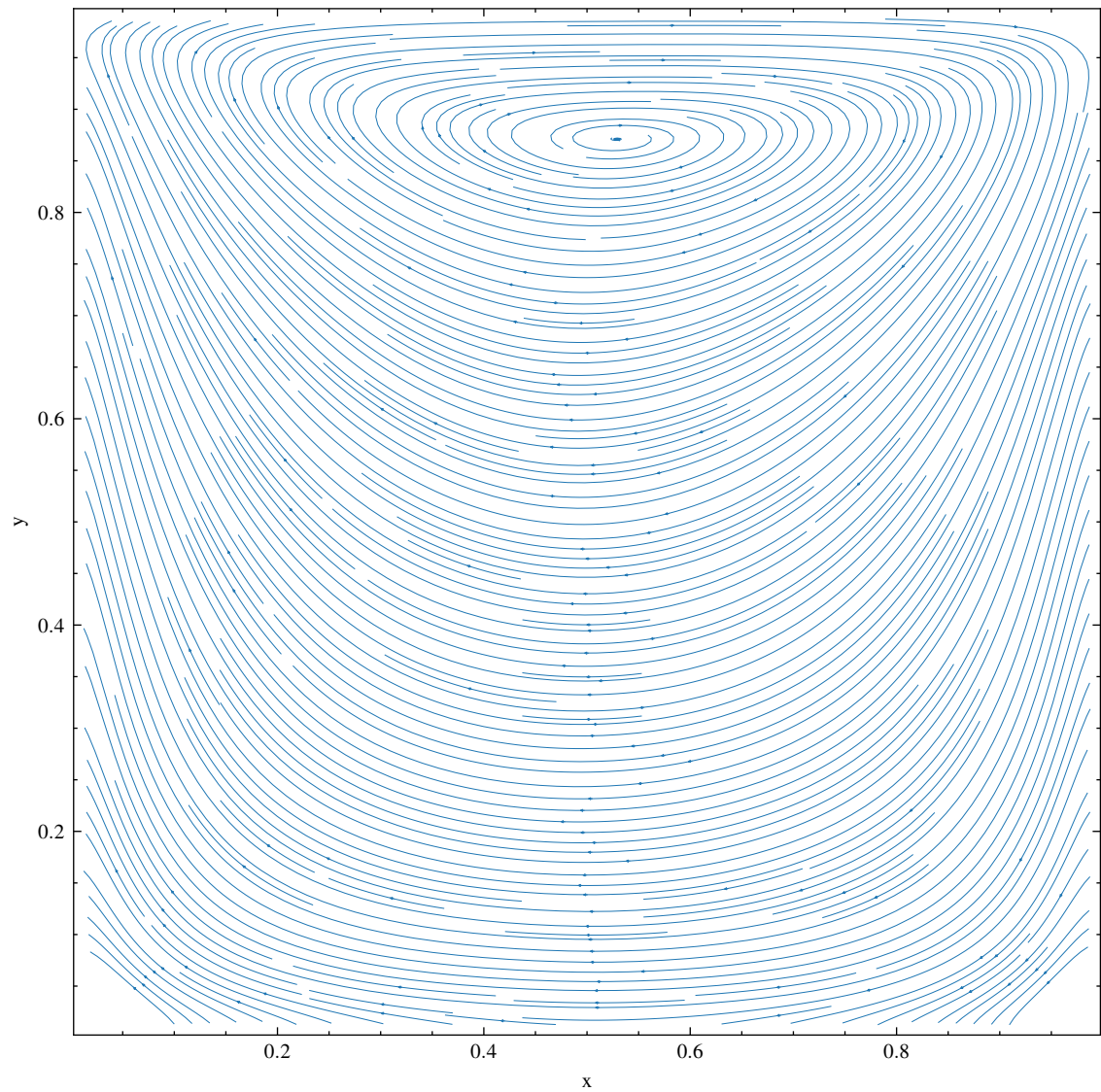
Streamlines — Simulation ID: 6013a033
