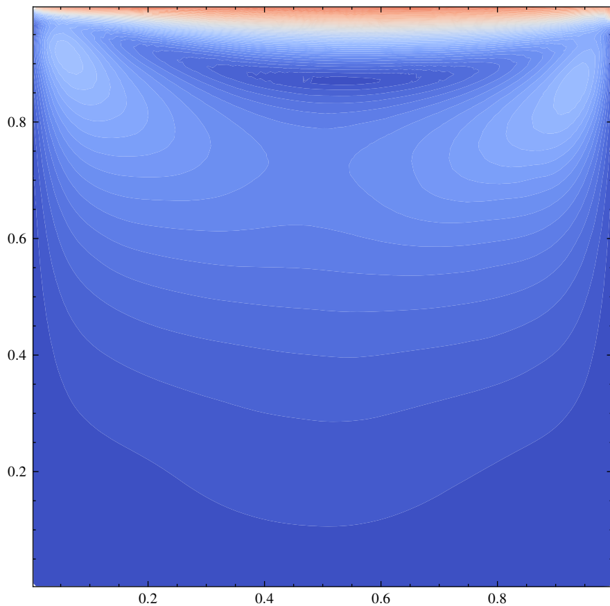
Velocity Magnitude — Simulation ID: 6013a033
