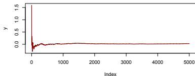
evolution de S_n en fonction de n : cas gaussien
