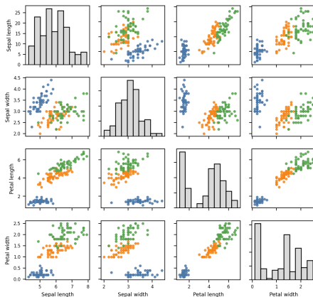
Matrice de nuages de points
