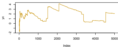
evolution de S_n en fonction de n : cas cauchy
