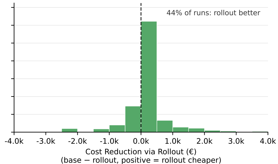
DB
