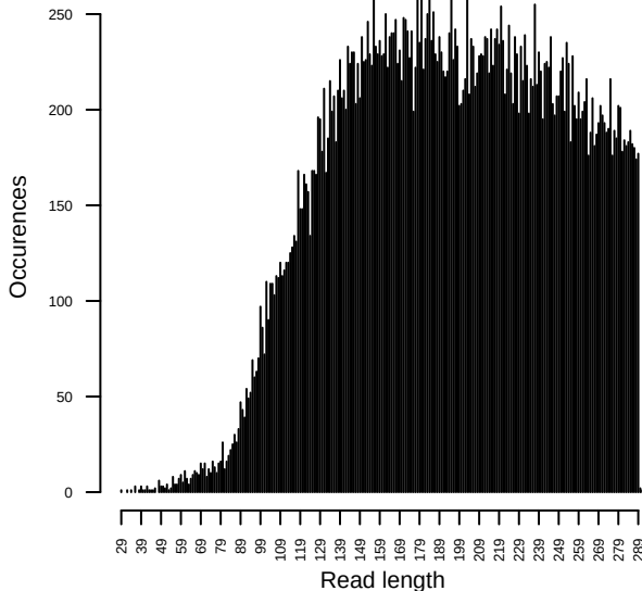
C>T
