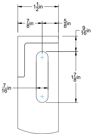
DETAIL N: Typ. Slot SCALE 1:2
