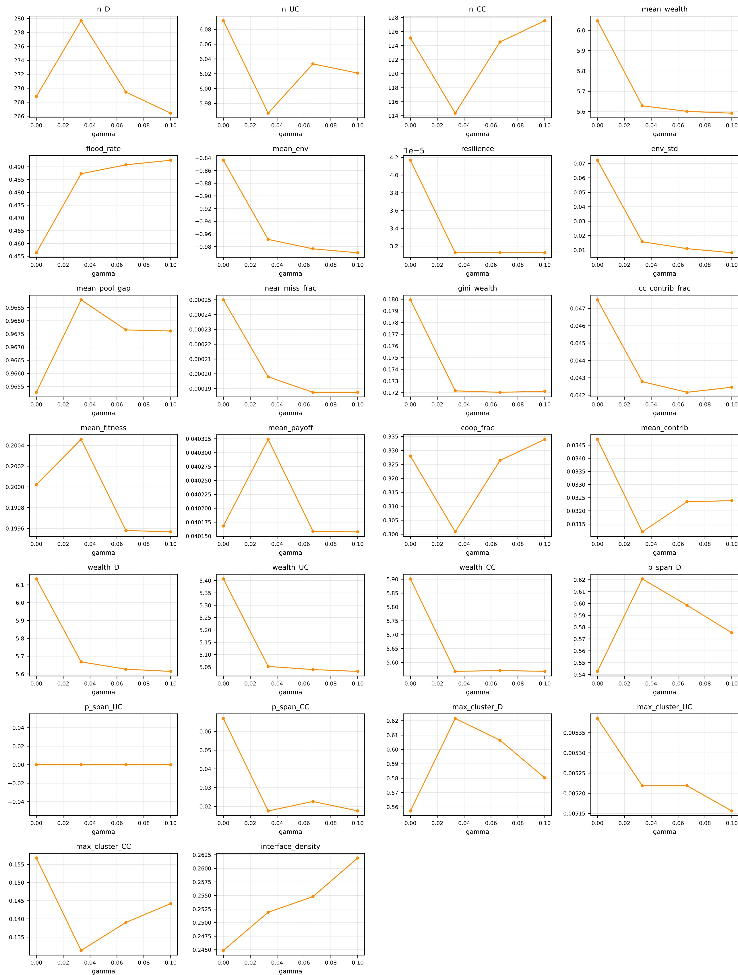
Order parameters vs gamma
