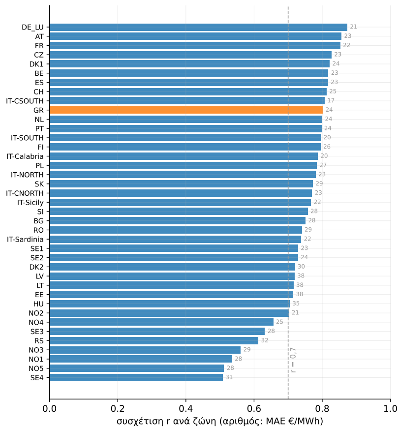
Σχήμα 5.11: Συσχέτιση ανά ζώνη στο πλήρες αρχείο cv37 (786 ημέρες): ο αριθμός δεξιά κάθε ράβδου είναι το MAE της ζώνης σε €/MWh. Με πορτοκαλί η ελληνική ζώνη.
