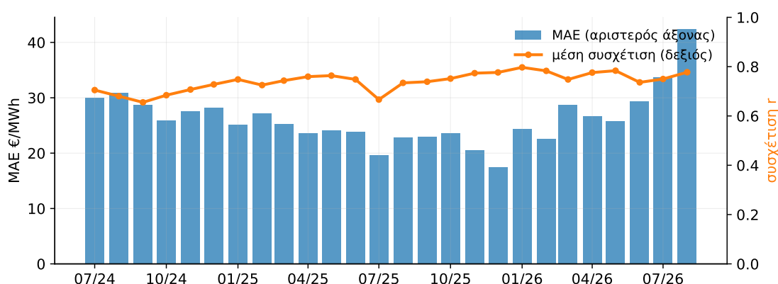
Σχήμα 5.10: Το αρχείο cv37 μήνα προς μήνα (7/2024–8/2026, 39 ζώνες): MAE αποτυπώματος (ράβδοι) και μέση συσχέτιση ανά ζώνη (γραμμή). Η συσχέτιση κρατιέται στο 0,7–0,8 σε όλο το παράθυρο· ο Αύγουστος του 2026 επιβαρύνεται από γνωστή διακοπή των D–1 εισόδων στην πηγή (λογαριασμός ENTSO-E), όχι από το μοντέλο.
