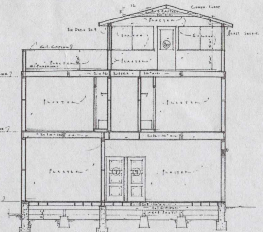
SECTION D-D SCALE 1/4\"/>
