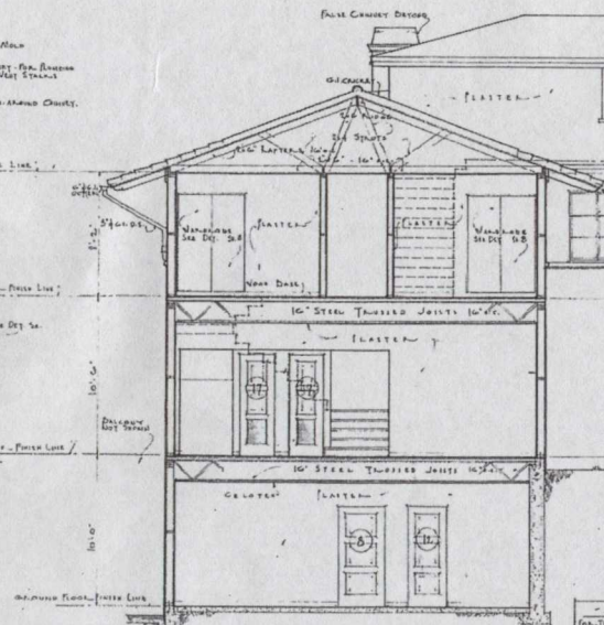
SECTION D-D SCALE 1/4\"/>
