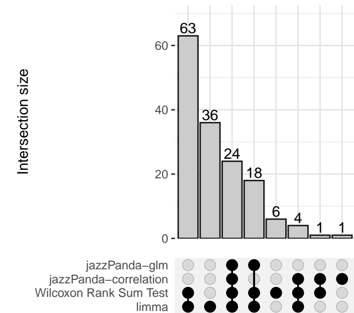
Endo_Blood
