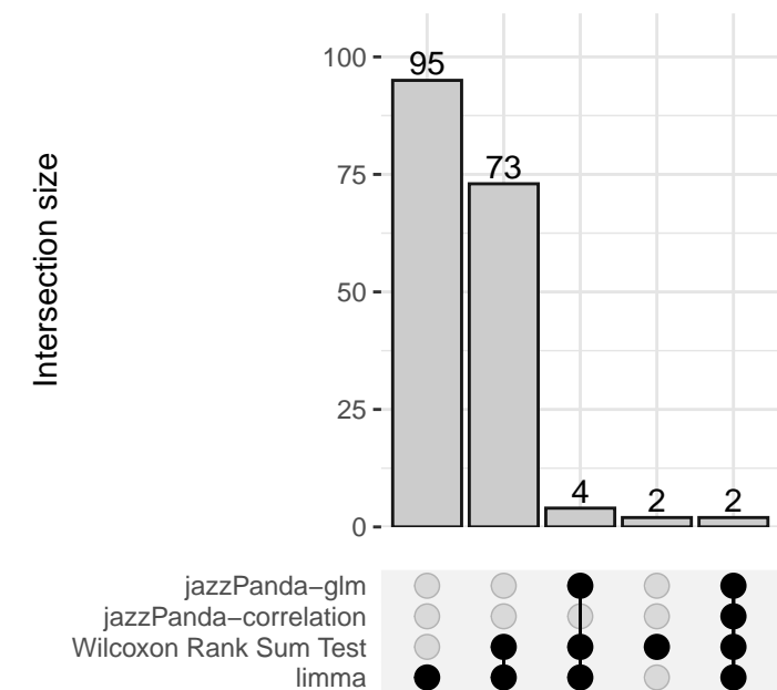
DC_Langerhans_cDC2
