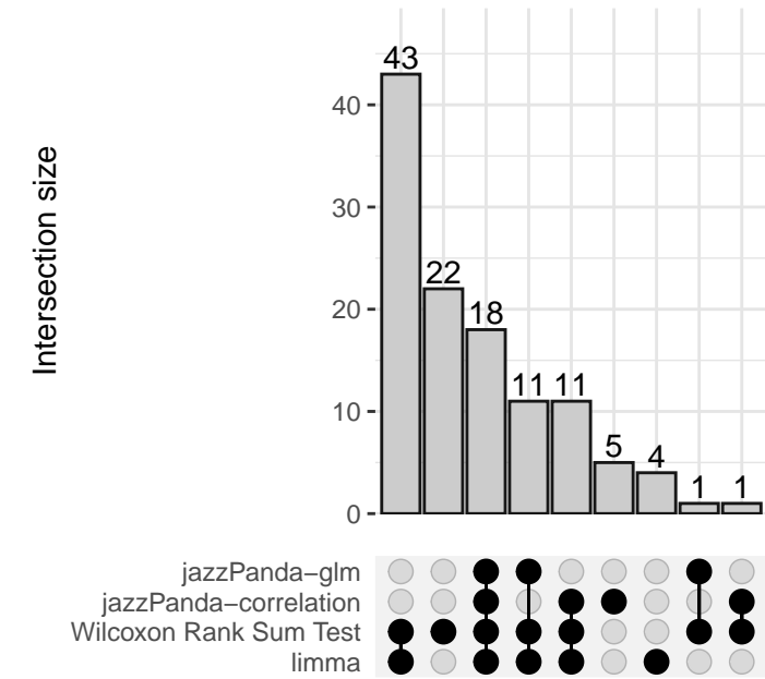
TAM_SPP1
