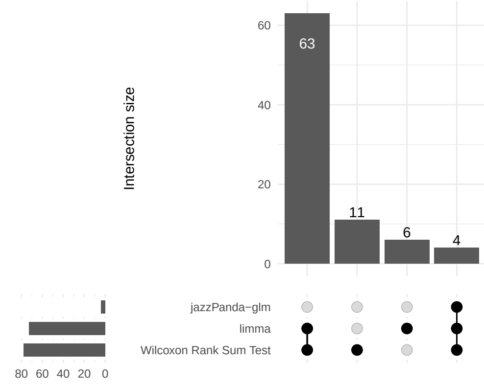
Dendritic
