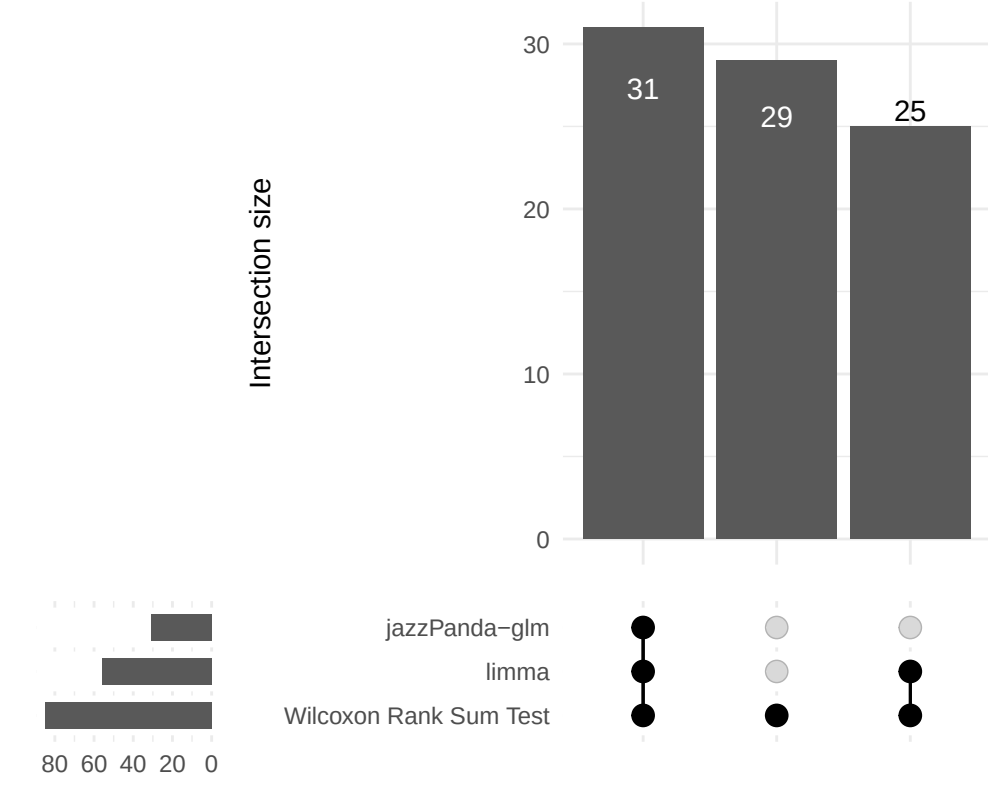
T_Cells
