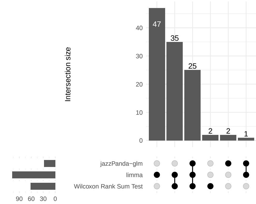
Stromal
