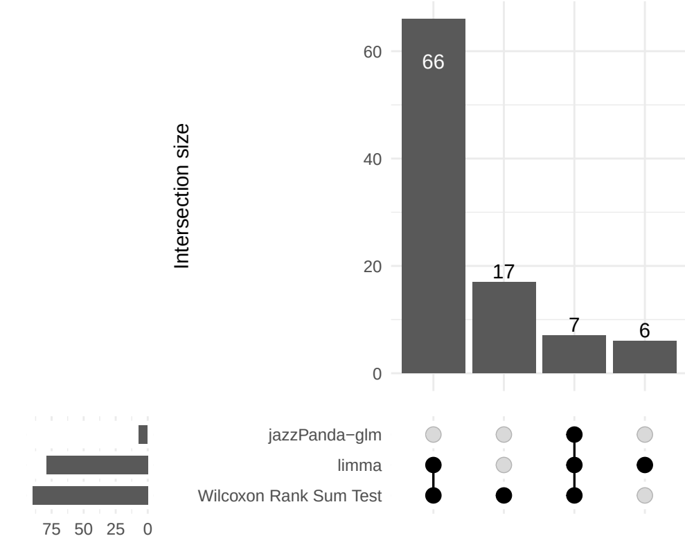
B_Cells
