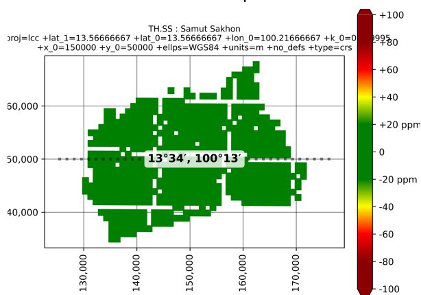
LDP Map
