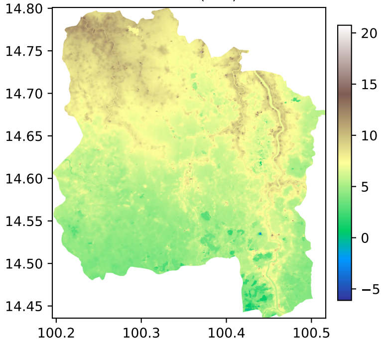
FABDEM (MSL)
