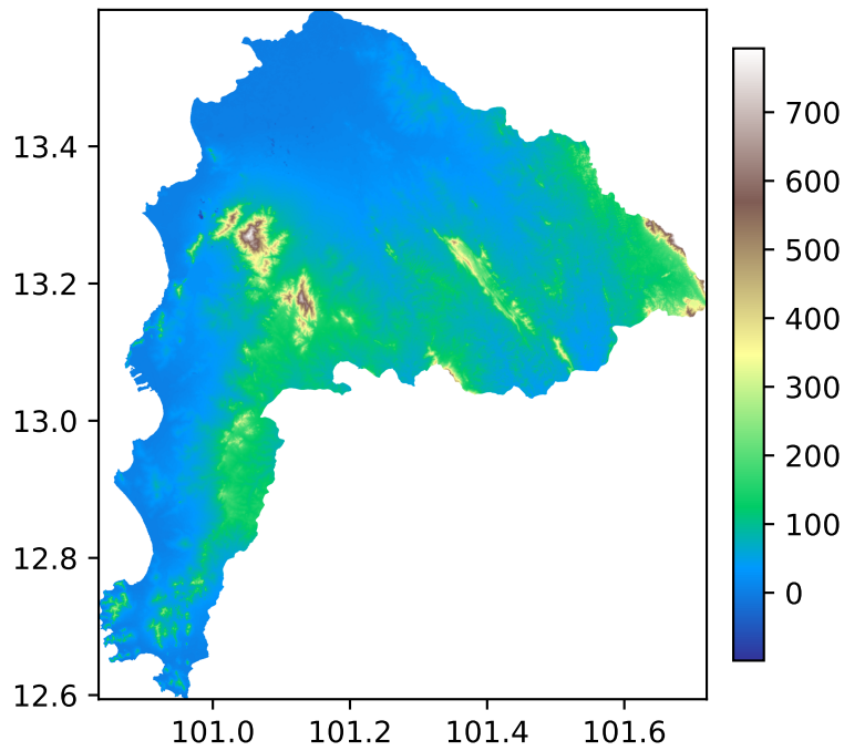
FABDEM (MSL)
