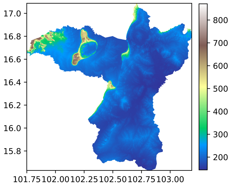
FABDEM (MSL)
