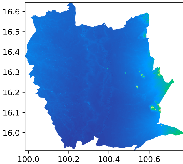
FABDEM (MSL)
