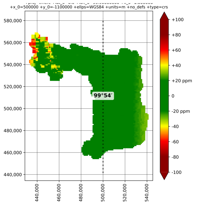
LDP Map
