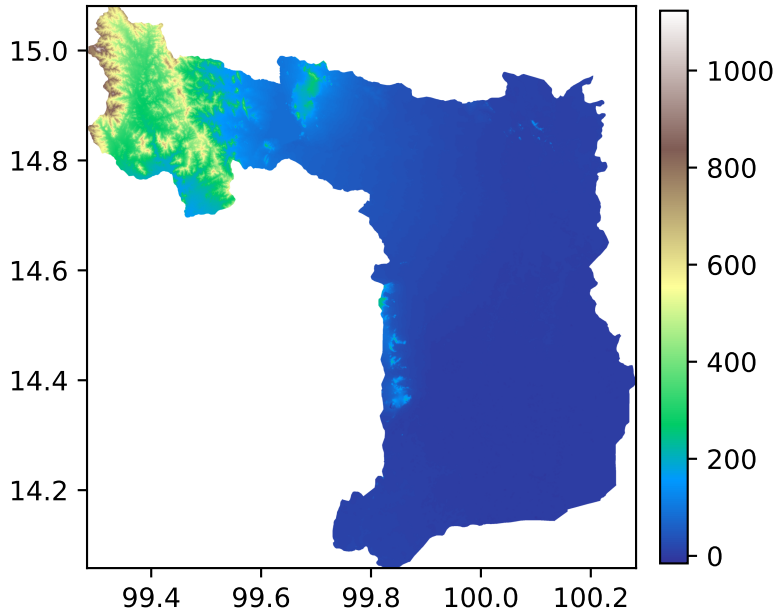
FABDEM (MSL)
