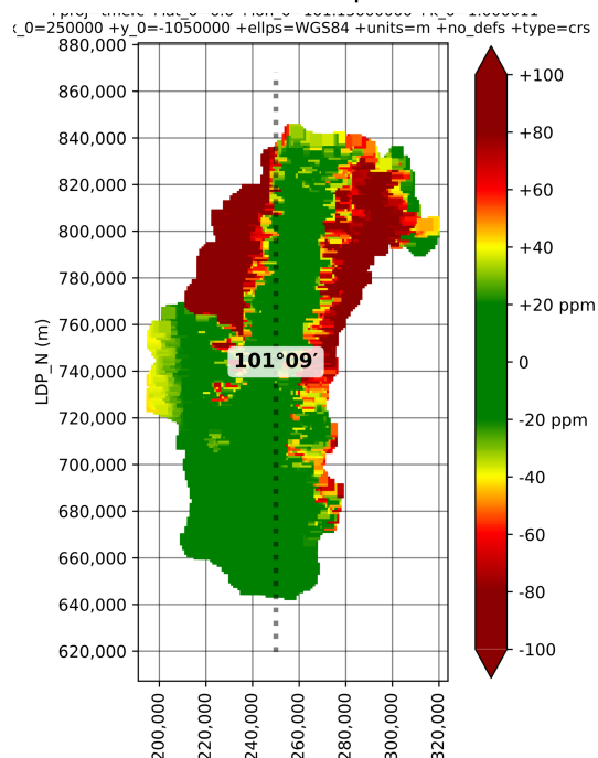
LDP Map
