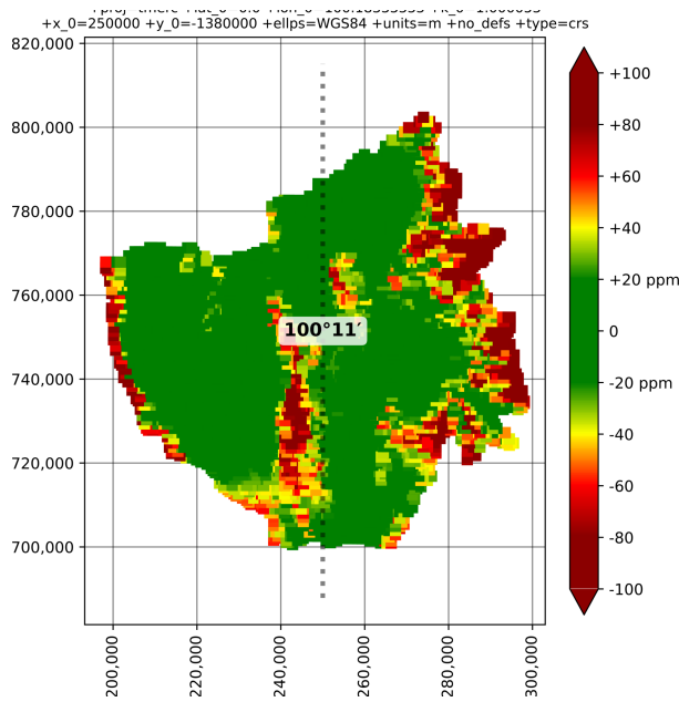
LDP Map
