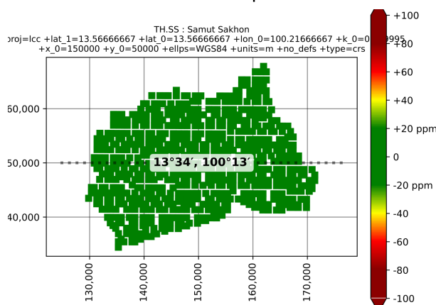
LDP Map
