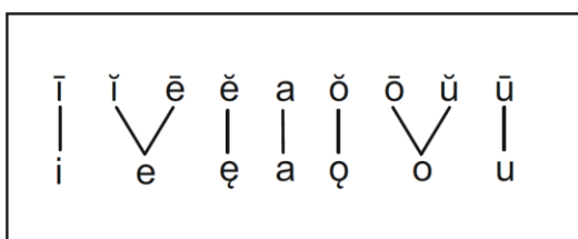
Abb. 1: Quantitätenkollaps
