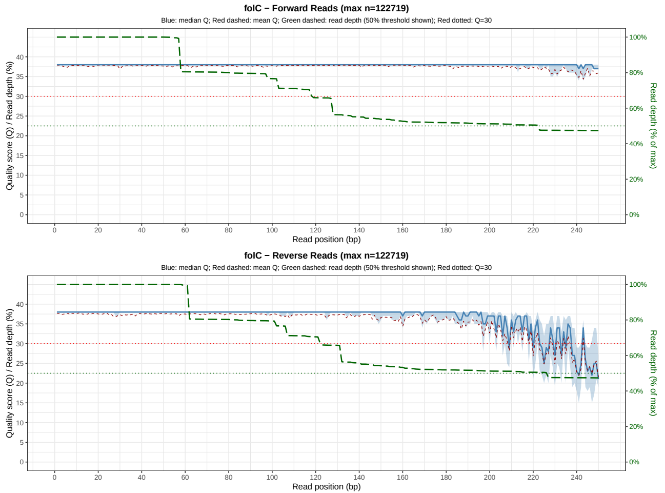
Рис.4.3. Агрегированный профиль качества ридов для гена folC . Верхний график — прямые риды, нижний — обратные риды. Голубая область — интервал между 25-м и 75-м процентилем качества; синяя сплошная линия — медиана качества; красная пунктирная линия — среднее качество; зеленая пунктирная линия — доля образцов, представленных на данной позиции. Горизонтальная красная пунктирная линия обозначает пороговое значение Q = 30 .
