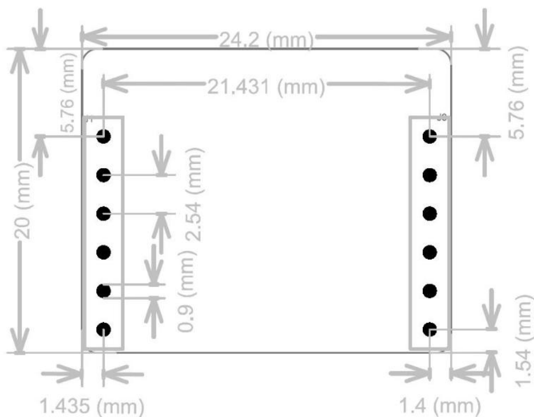
图 3 MINI 核心板尺寸图
