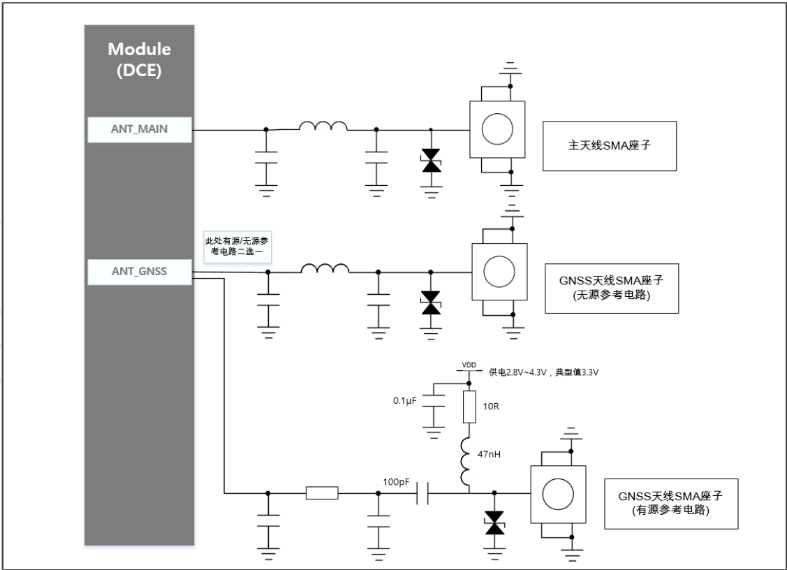
Figure 17. 射频参考电路
