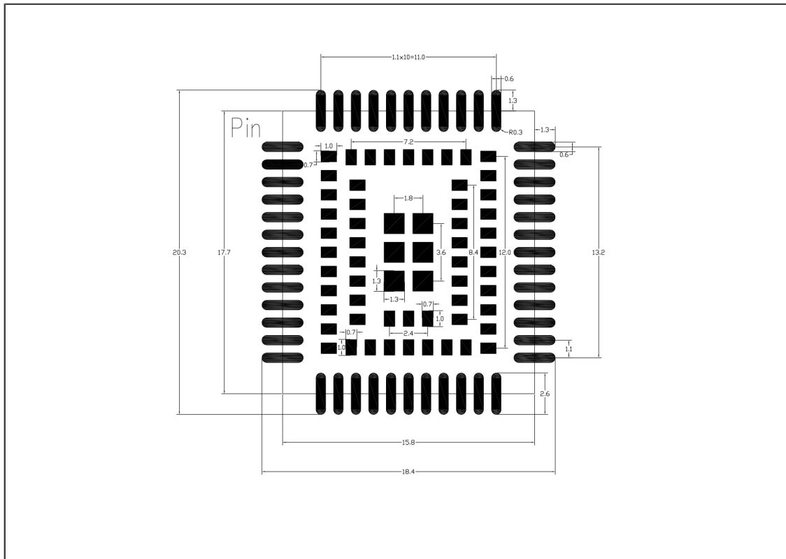
Figure 20. PCB推荐封装 (单位: mm)
