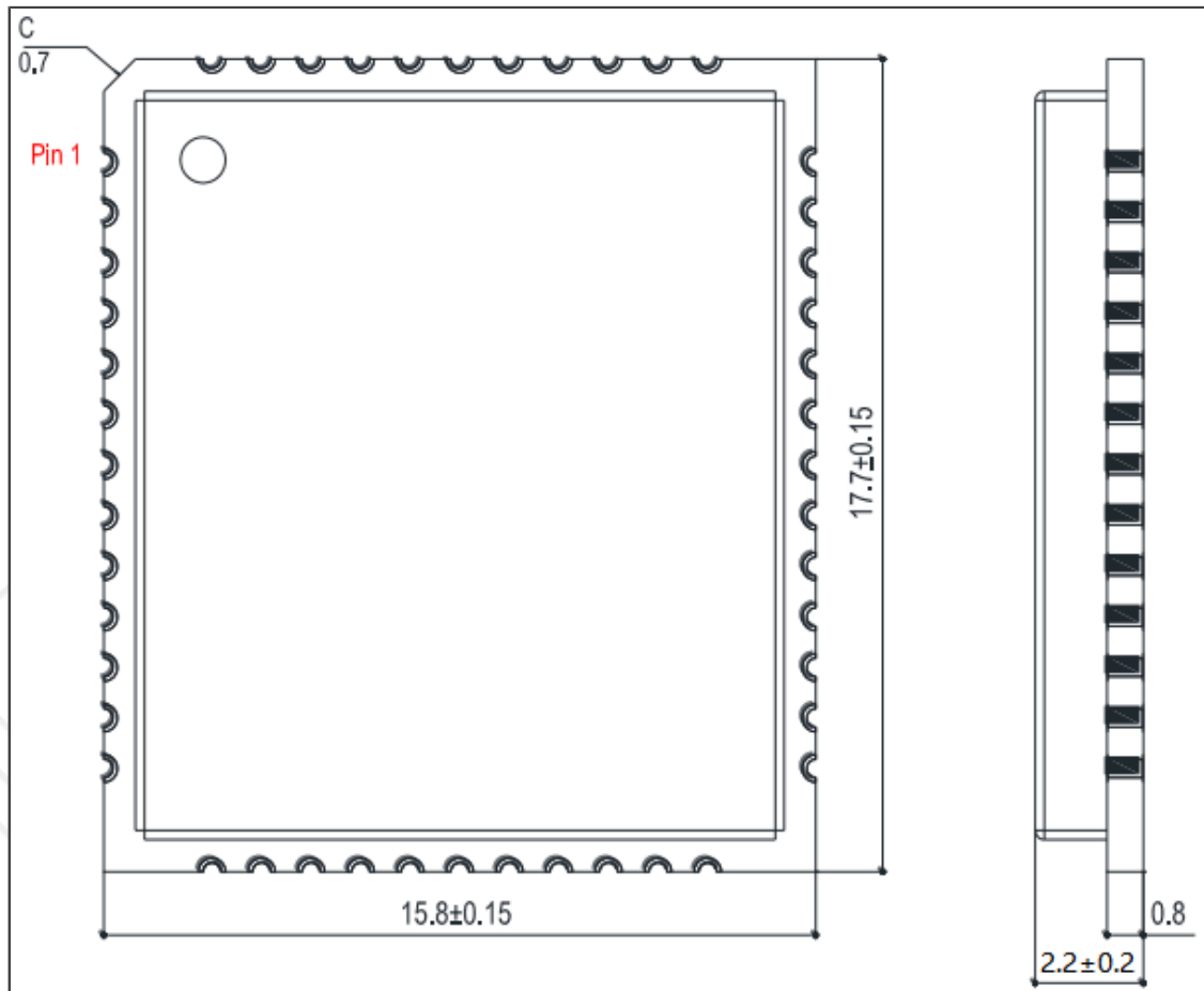
Figure 18. 模组顶视图（单位：mm）
