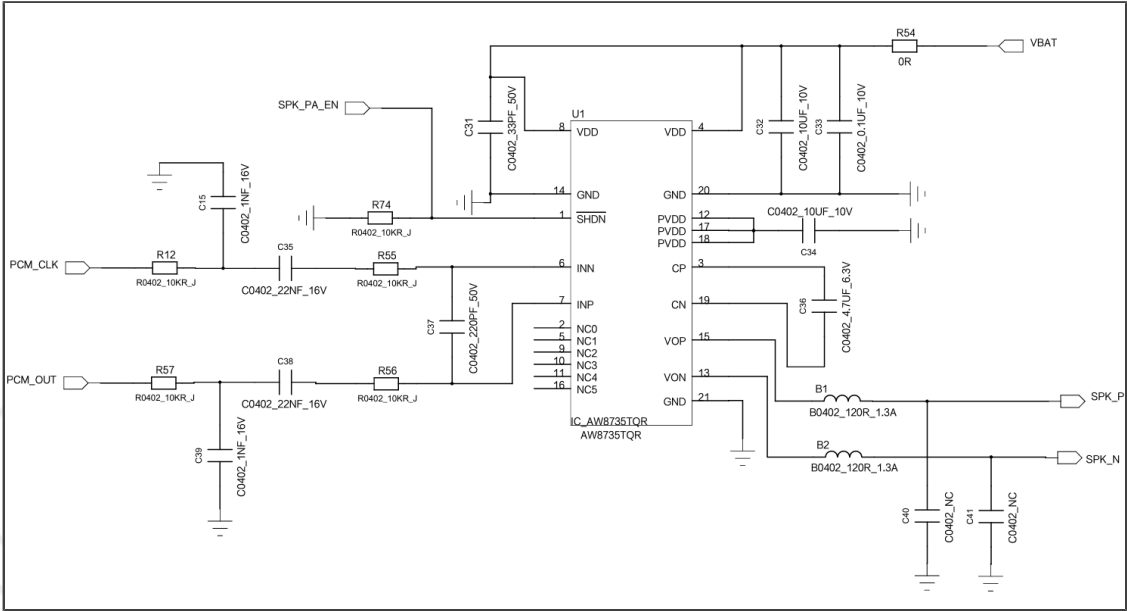
Figure 9. PWM方案参考设计
