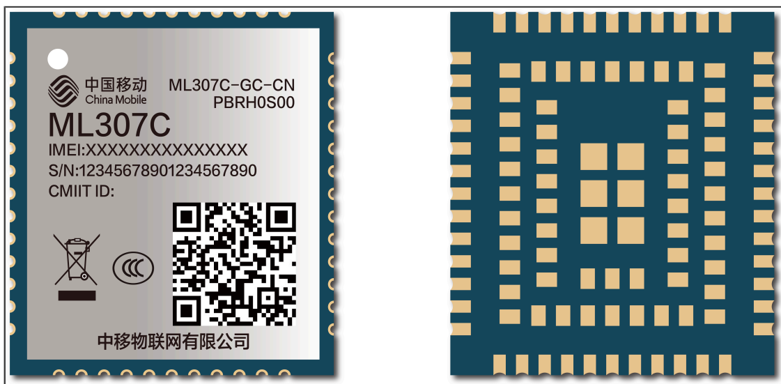
Figure 1. 模组示意图
