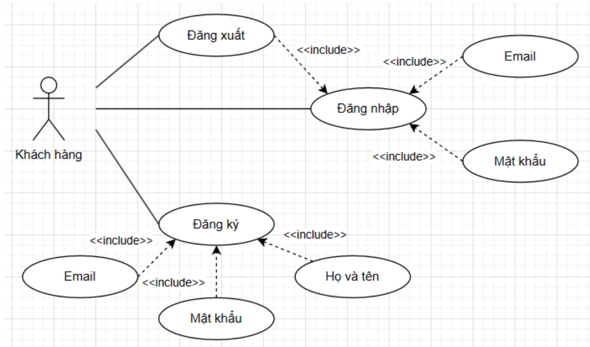
Hình 7: Sơ đồ usecase đăng ký và đăng nhập
