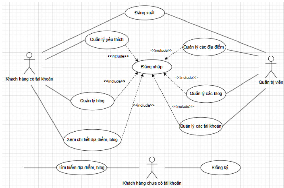
Hình 6: Sơ đồ usecase tổng quát
