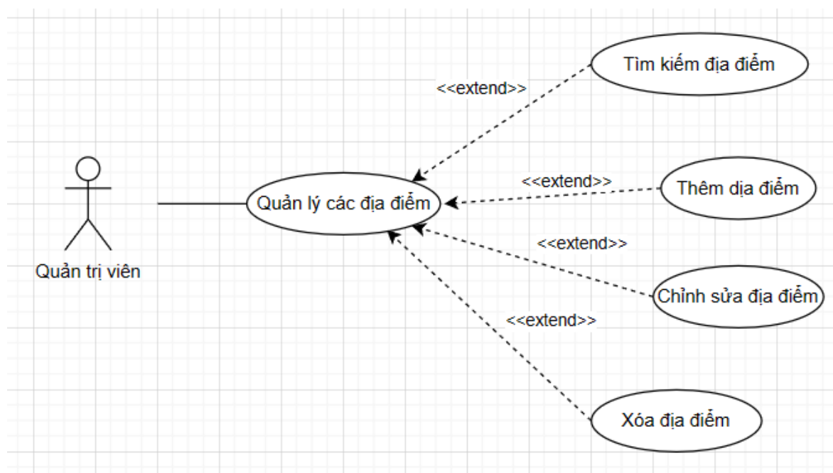
Hình 10: Sơ đồ usecase quản lý các địa điểm
