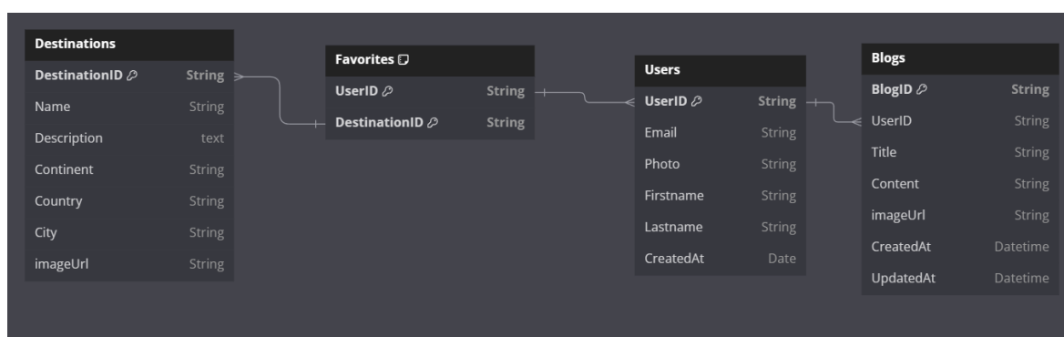
Hình 13: Mô hình CDM
