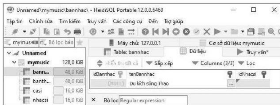
Hình 22.2. Minh họa thao tác nhập dữ liệu
