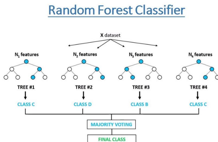
รูปภาพที่ 18 การจำแนก Random Forest
