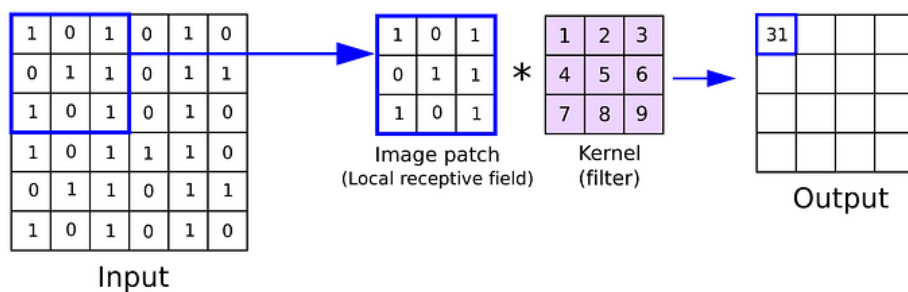
รูปภาพที่ 10 ตัวกรอง
