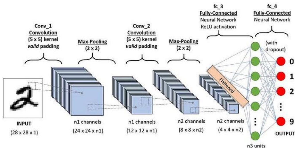
รูปภาพที่ 9 Convolutional Neural Network
