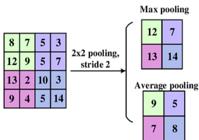
รูปภาพที่ 13 Pooling Layer
