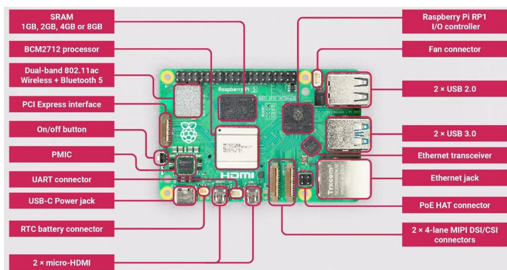
รูปภาพที่ 3 ส่วนประกอบสำคัญ Raspberry Pi 5
