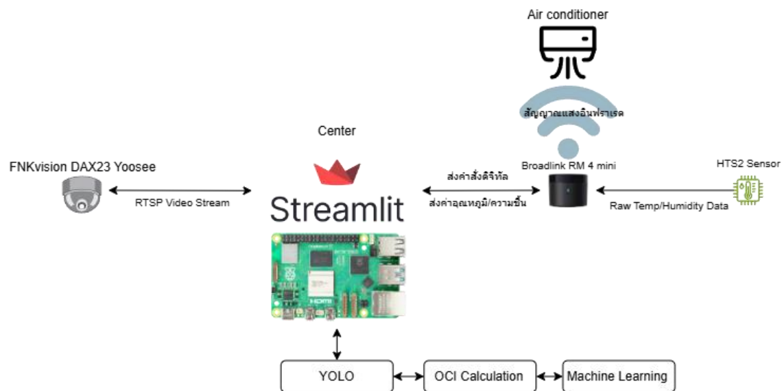
รูปภาพที่ 25 แผนภาพแสดงการไหลของข้อมูลและการควบคุม
