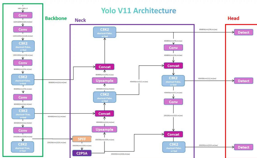
รูปภาพที่ 16 YOLOv11 Architecture
