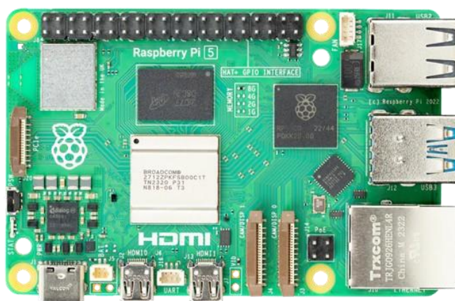
รูปภาพที่ 2 Raspberry Pi 5
