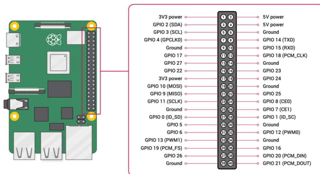
รูปภาพที่ 4 พอร์ต GPIO Raspberry Pi 5
