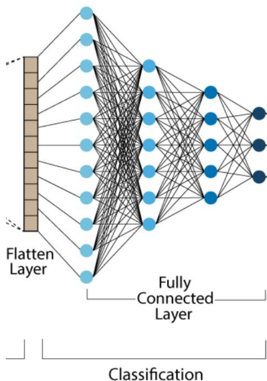
รูปภาพที่ 15 Fully-Connected Layer
