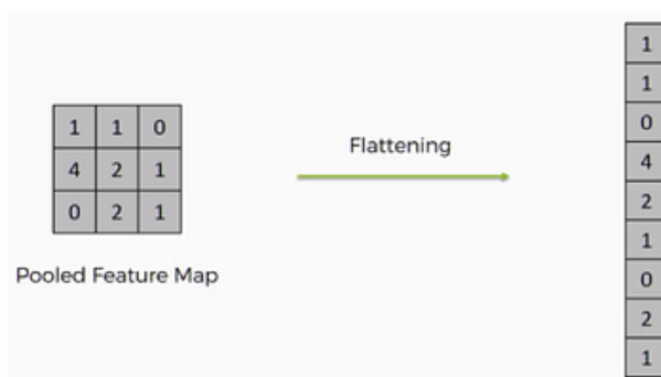
รูปภาพที่ 14 Flattening
