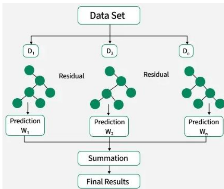
รูปภาพที่ 19 การจำแนก Extreme Gradient Boosting
