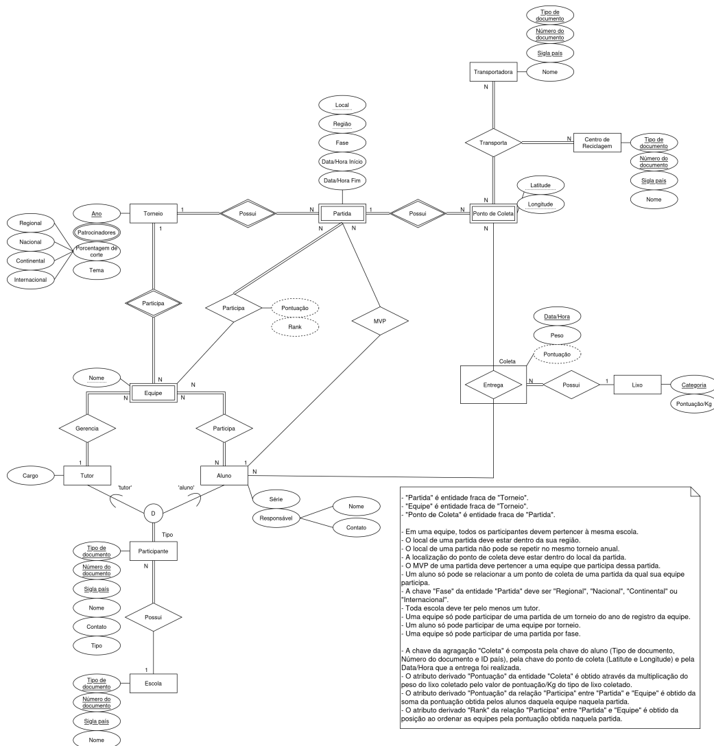
Figura 2: Diagrama do Modelo Entidade-Relacionamento
