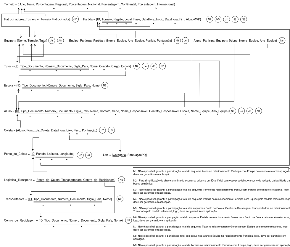
Figura 3: Mapeamento do MER da Figura 2 para o Modelo Relacional
