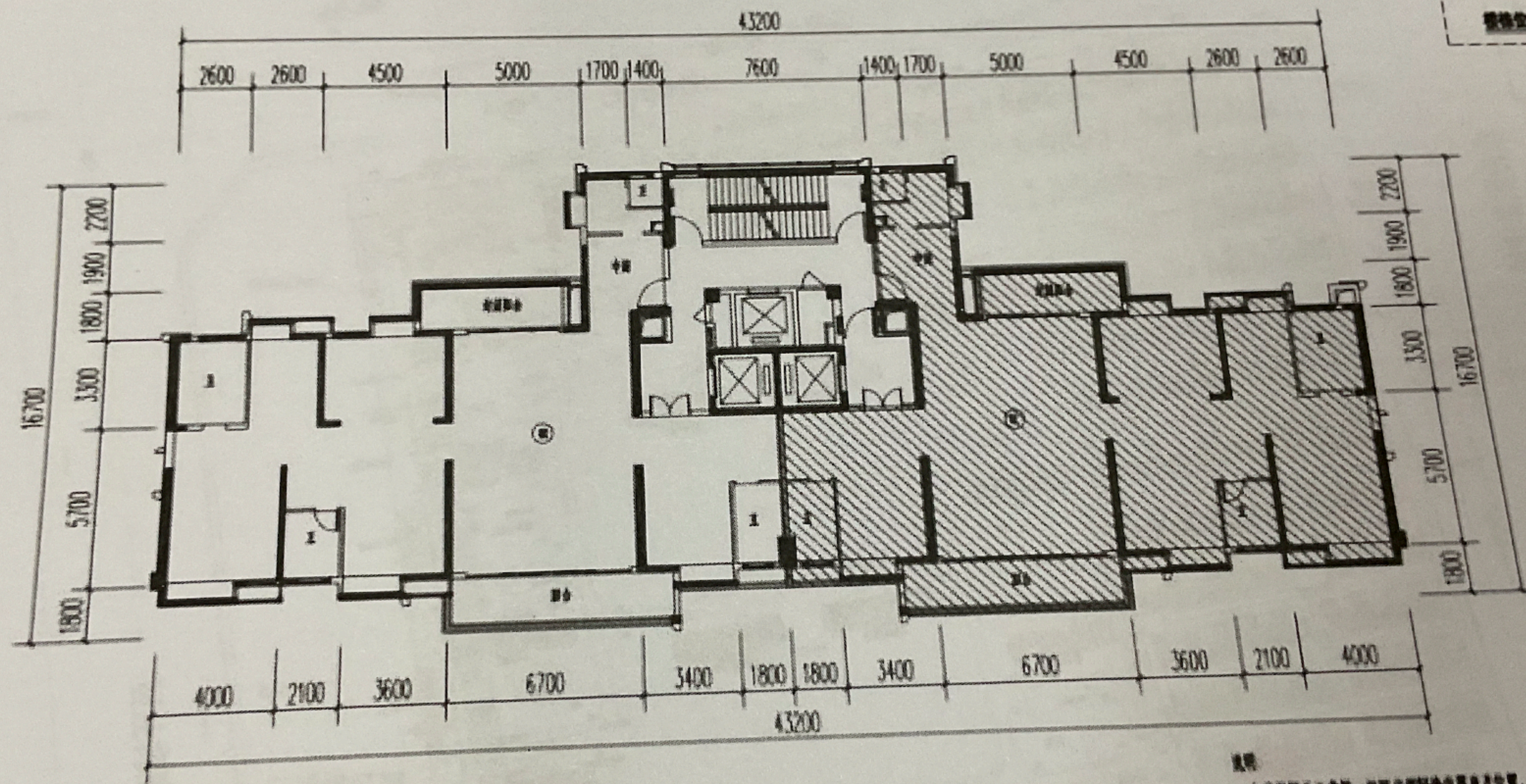
5#楼四~二十九层平面图
