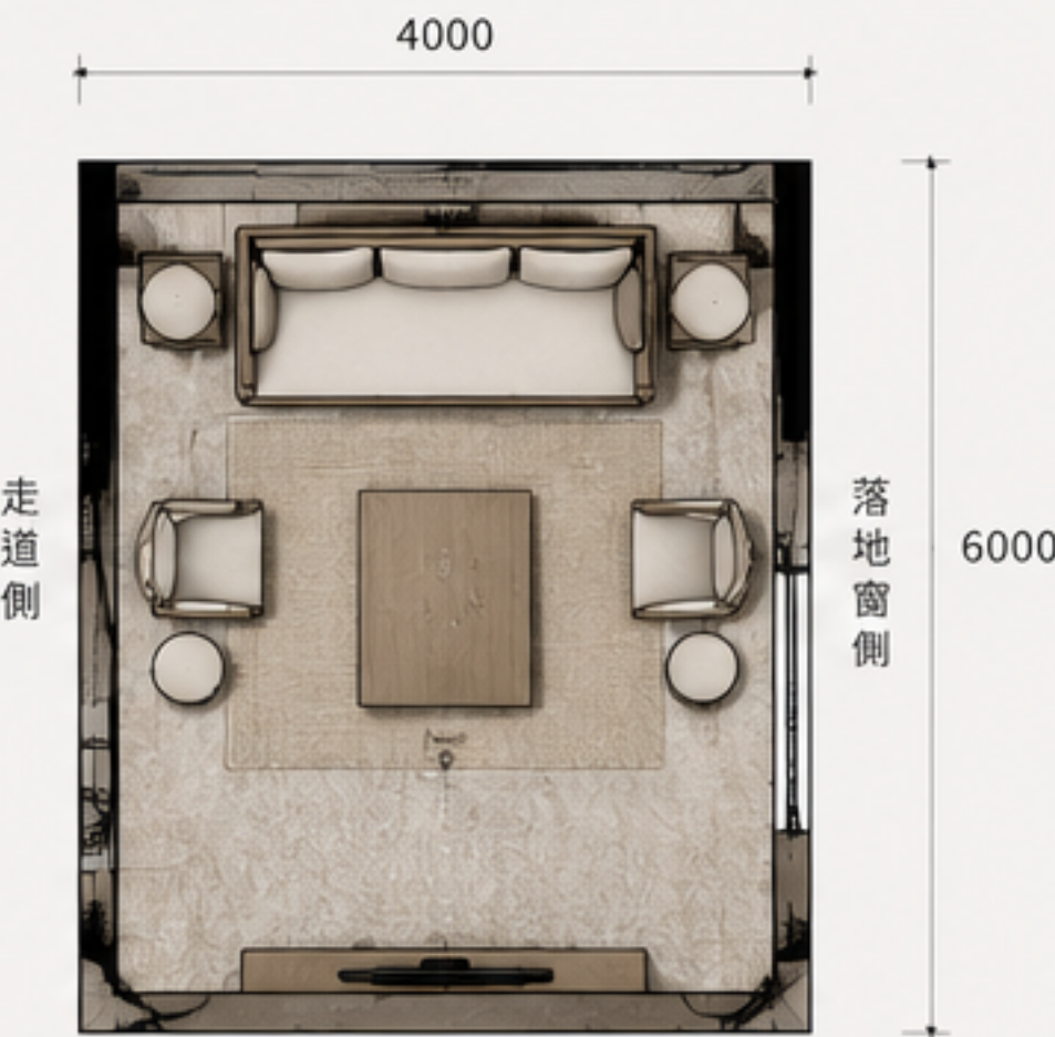
平面配置圖（單位：mm）
