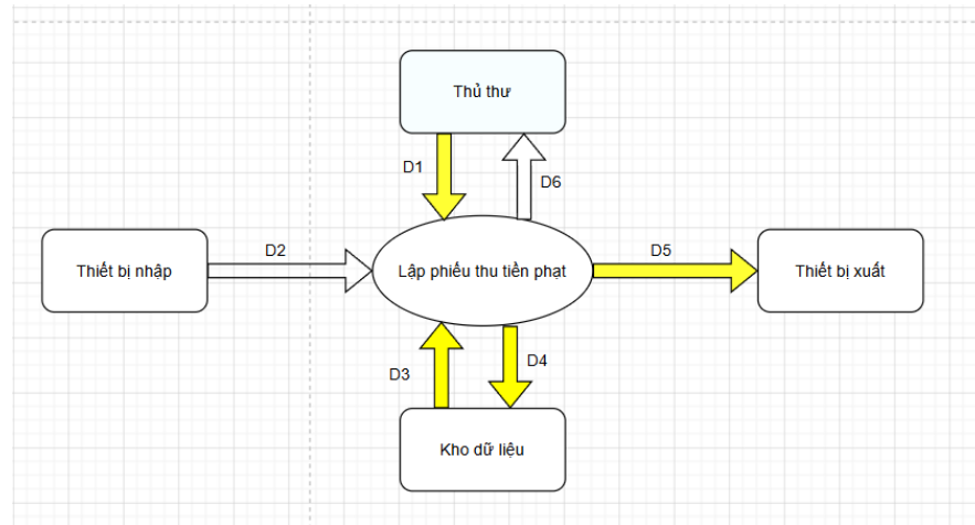
Hình 7. Sơ đồ luồng dữ liệu công việc Lập phiếu thu tiền phạt
