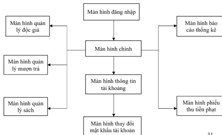
Hình 20. Sơ đồ liên kết các màn hình
