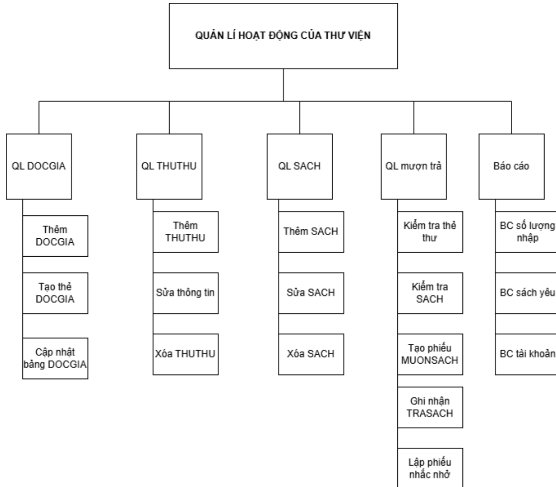
Hình 1. Mô hình tổng thể của hệ thống
