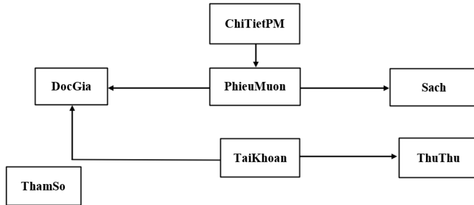
Hình 19. Sơ đồ logic hoàn chỉnh
