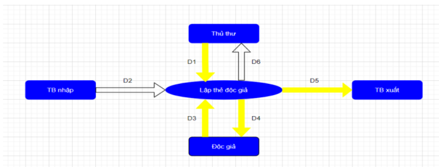
Hình 2. Sơ đồ luồng dữ liệu cho thẻ độc giả
