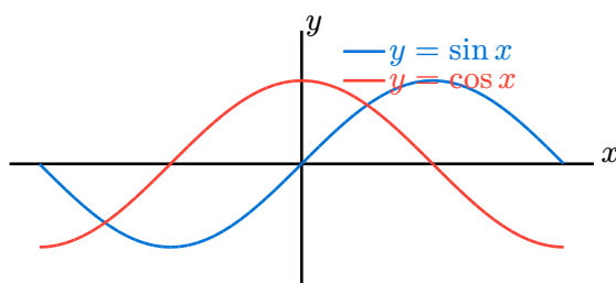
Figure 5: Đồ thị y = \sin x (xanh) và y = \cos x (đỏ) trên đoạn [-\pi, \pi]
