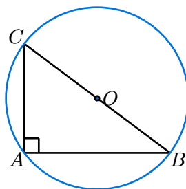
Figure 4: Tam giác vuông ABC và đường tròn ngoại tiếp — tâm O là trung điểm BC
