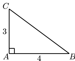
Figure 3: Tam giác vuông ABC với ký hiệu góc vuông tại A
