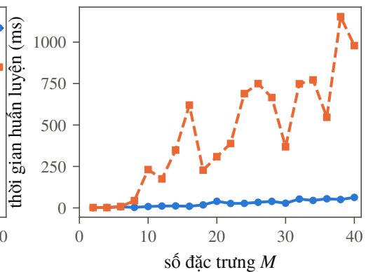
(d) Thời gian huấn luyện theo M
