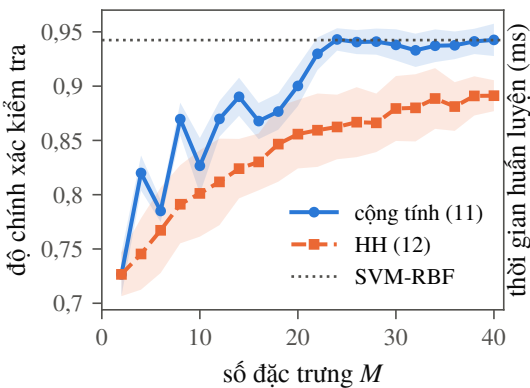
(c) Độ chính xác theo M
