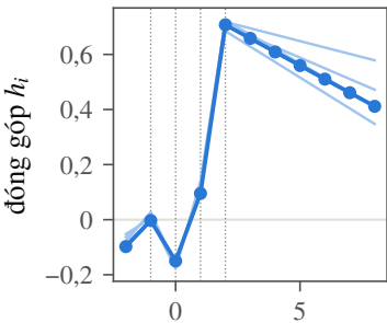
PAY_0 (tháng 9)
