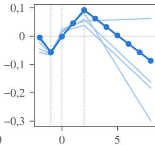
PAY_2 (tháng 8)
