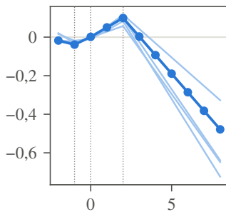
PAY_4 (tháng 6)
