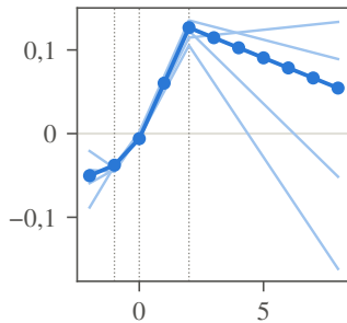
PAY_3 (tháng 7)
