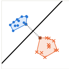
(c) hai bao lồi
