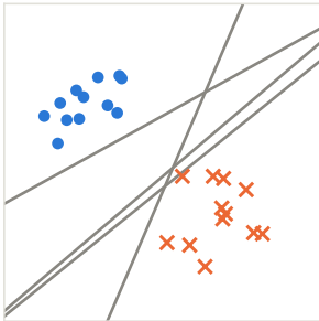
(a) nhiều biên tách được
