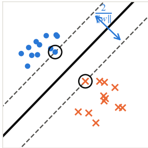
(b) lề cực đại
