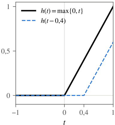
(a) Hàm bản lề (ReLU)
