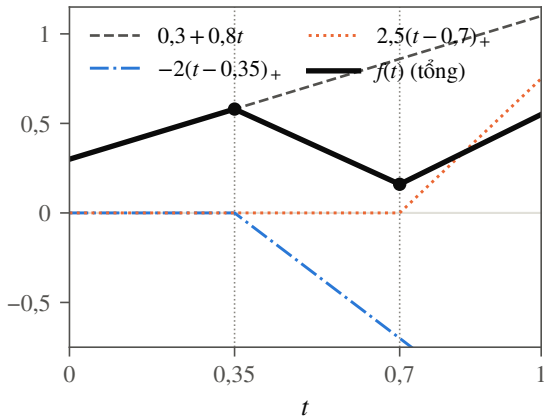
(b) Hàm PWL một biến = phần affine + các bản lề
